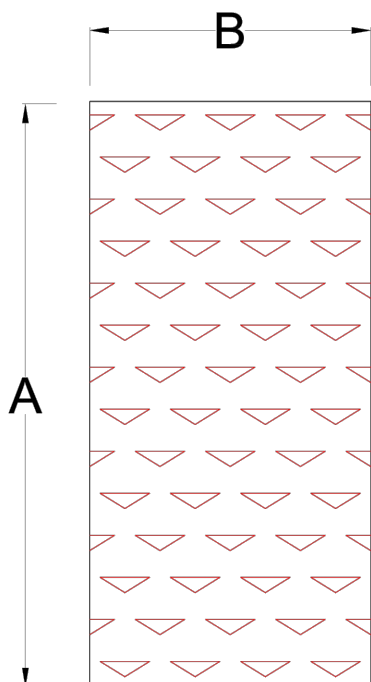
Schema d'orditura del pannello
